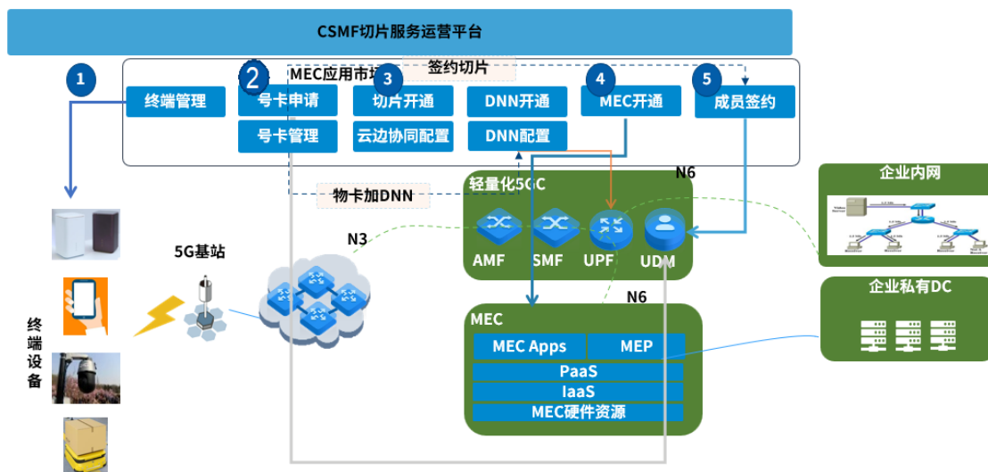
图6-4 融合切片业务端到端支撑
